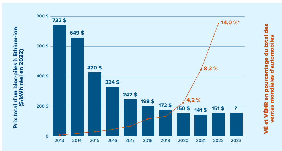
FIGURE 1 – APRÈS UNE DÉCENNIE DE DÉFLATION DU PRIX DES BATTERIES, LES COÛTS ONT AUGMENTÉ EN 2022
